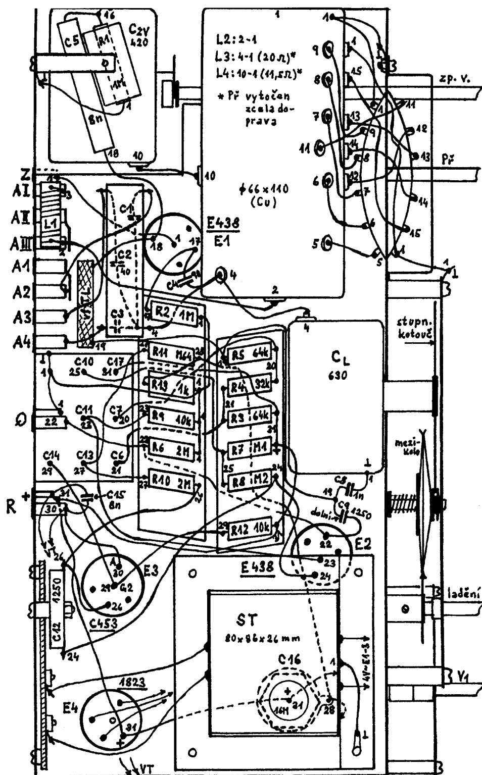
Obr. 2. Rozmístění součástek a vedení spojů pod šasi
